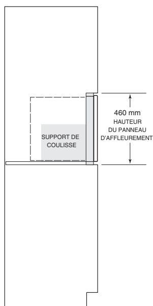
VUE LATÉRALE
