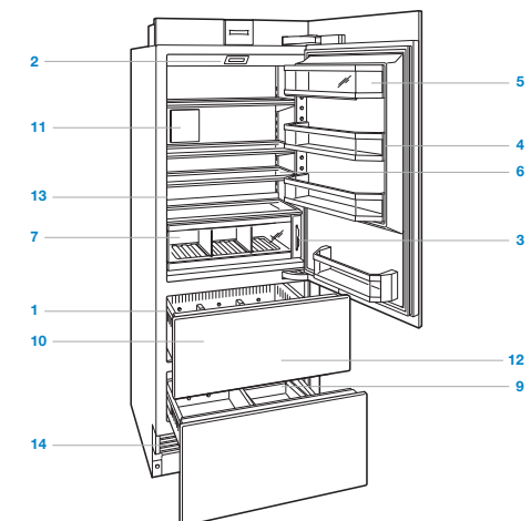
Hoge combinatie.
