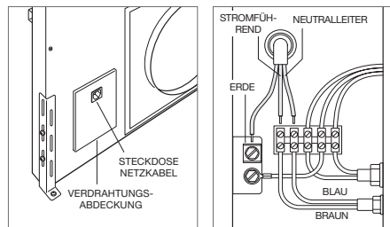
Verdrahtungsort.
