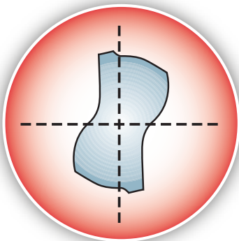
Parabelförmige Spannut
